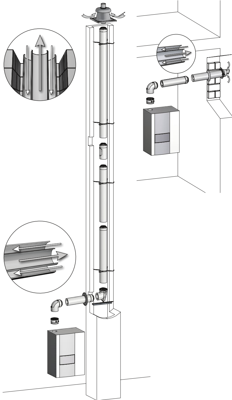
Schachtsystem konzentrisch
